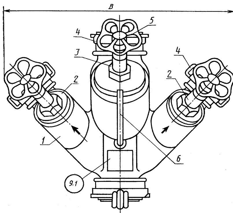
Трехходовое разветвление
