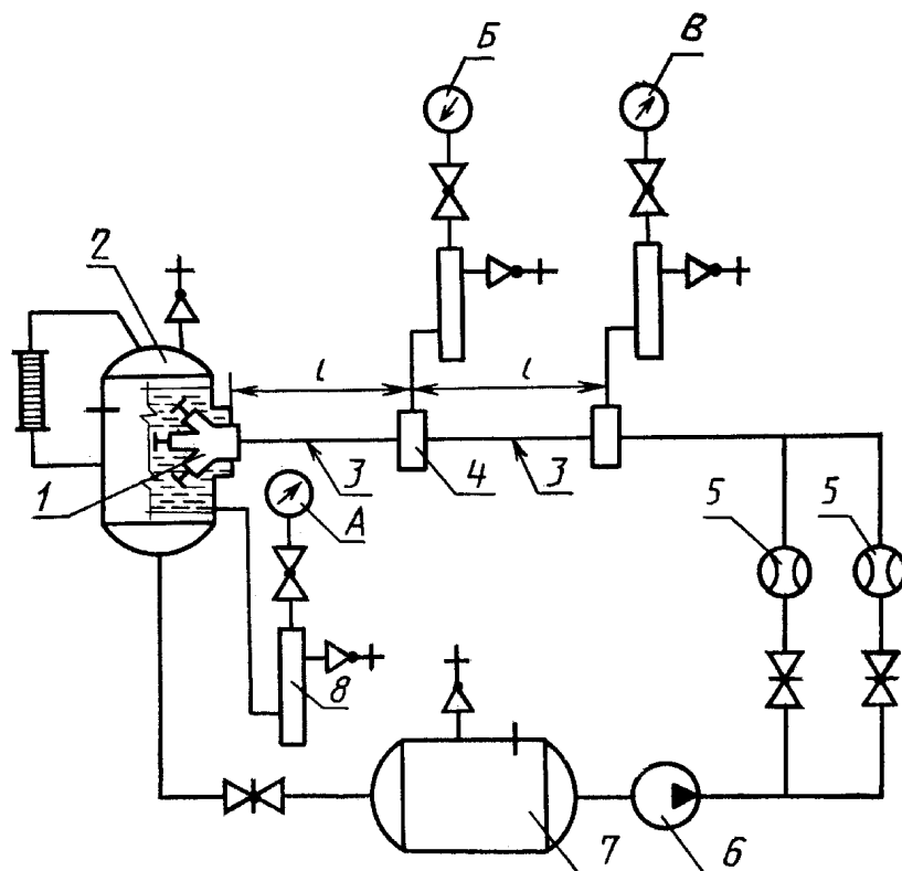
Схема стенда для проверки коэффициента гидравлического сопротивления
