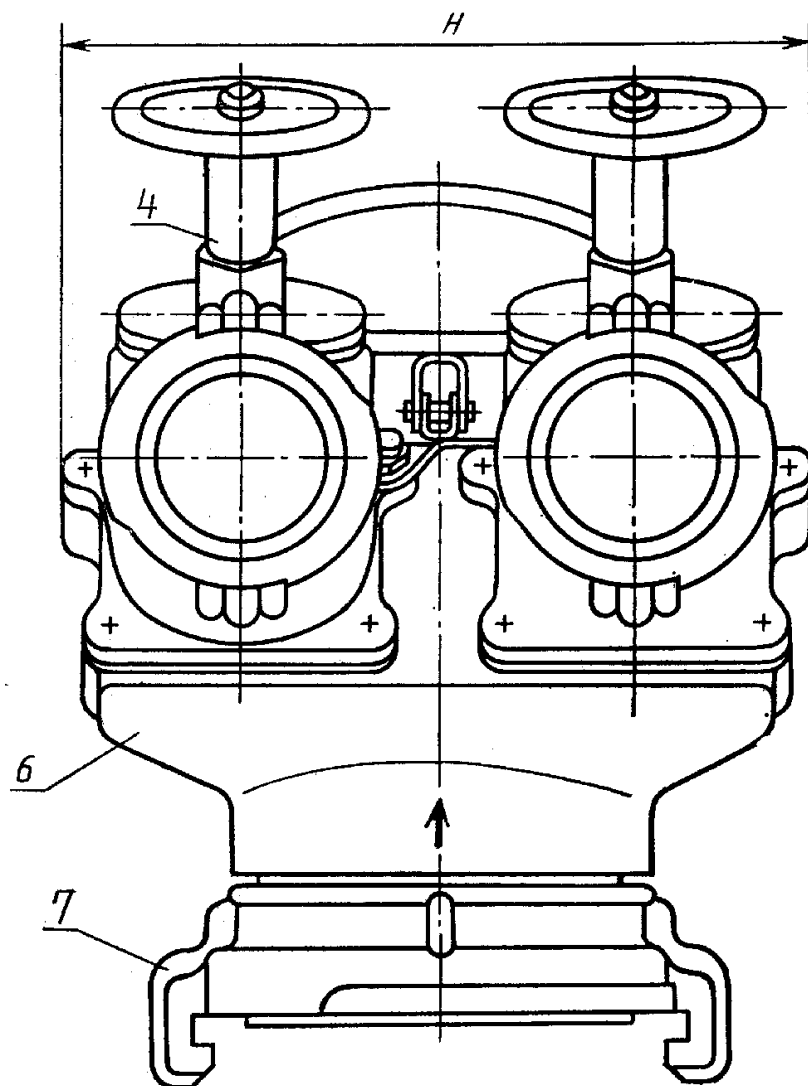
1—ручка, 2—маховик, 3—соединительная головка на выходном патрубке, 4—перекрывающее устройство, 5—затворный клапан, 6—корпус, 7—соединительная головка на входном патрубке
